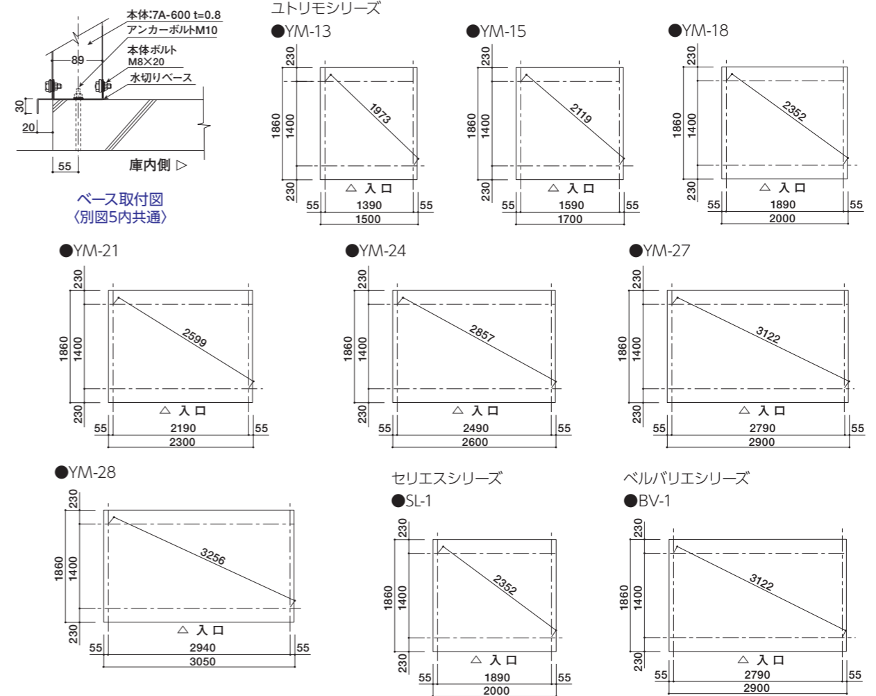
別図5 ■カスケード物置(単位mm)
