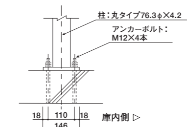
ベースプレート取付図
