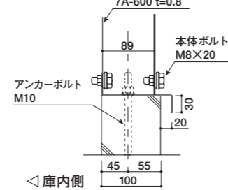
ベース取付図
