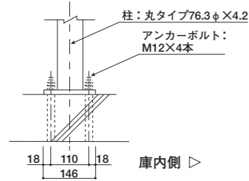
ベースプレート取付図
