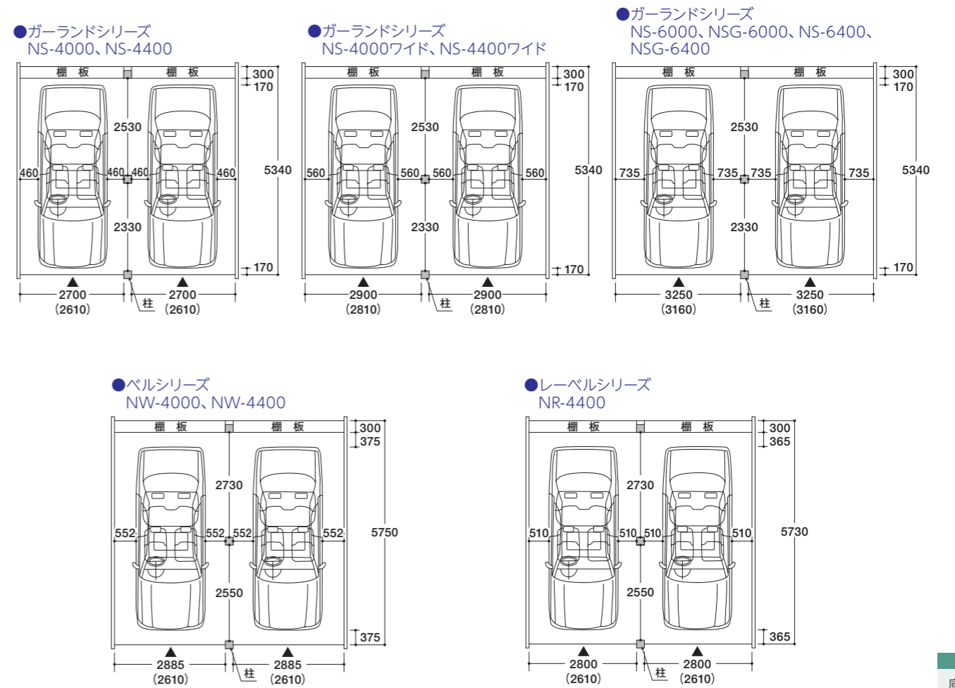
別図2 ■カスケードガレージ(連棟) (単位mm) ※( )内は有効開口幅です。
