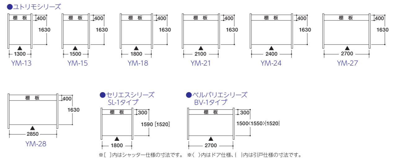
別図3 ■カスケード物置 (単位mm) カスケード物置 庫内スペース参考例
