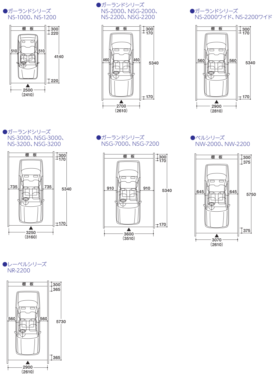
別図1 ■カスケードガレージ(単棟) (単位mm) ※( )内は有効開口幅です。
